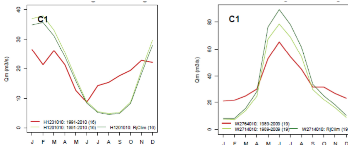
Figure 4 : Impact de grands réservoirs situés sur les cours d'eau, illustrés par la comparaison entre les débits amont (en vert) et aval (en rouge) : à gauche : sur l'Aube à Blaincourt, après deux retenues de 170 Mm 3 dédiées au soutien d'étiage, à droite : sur la Romanche à Bourg d'Oissan, après deux retenues de 183 Mm 3 dédiées à la production d'hydroélectricité. Figures issues de Cipriani et Sauquet (2014) 10
