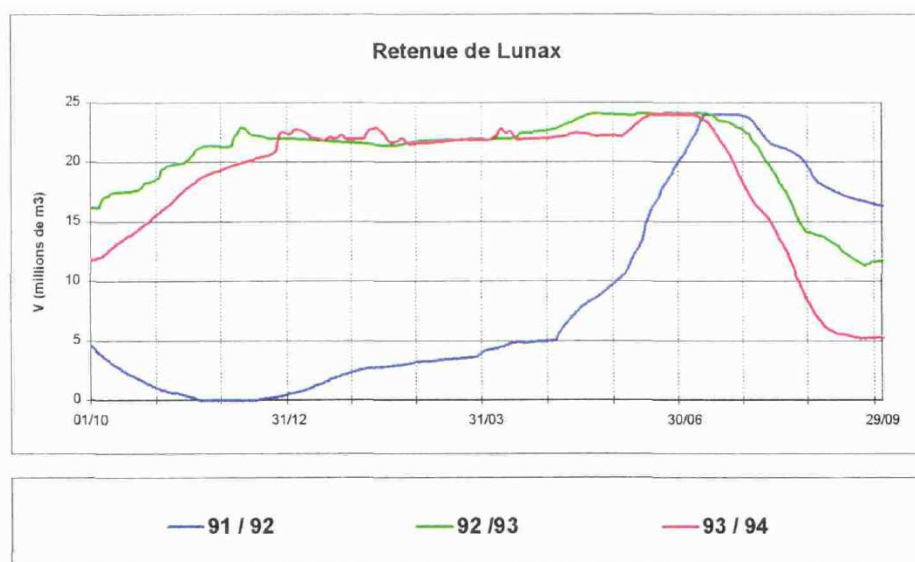
Figure 3 : Evolution du volume stocké dans une grande retenue Gasconne (Synthèse Piren, 1996 9 )
