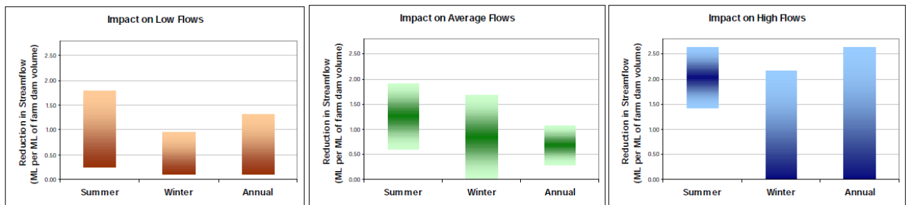
Figure 10 : Impacts des réseaux de retenues sur les débits des rivières en été, en hiver et en moyenne sur l'année. La différence de débit est rapportée à la capacité cumulée des retenues. A gauche l'impact sur les faibles débits, au milieu sur les débits moyens et à droite sur les forts débits. Les valeurs sont une compilation d'estimations faites par modélisation sur un ensemble de bassins versants dans la province de Victoria – Australie-
