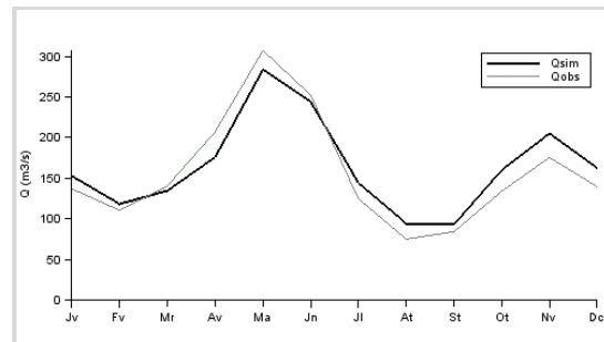
Fig. 3 Débits mensuels moyens observés ( Q_{obs} ) et naturels ( Q_{sim} ) à Cadarache.
