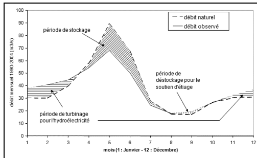
Fig. 2 Influence de la gestion des réserves d'eau sur le régime hydrologique naturel.
