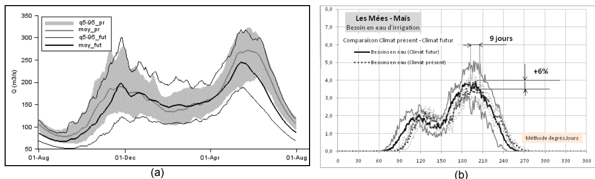
Fig. 4 Résultats de simulations temps présent et futur : débits naturels de la Durance à Cadarache (a) et besoins en eau d'irrigation du maïs (b) (moyenne d'ensemble en trait épais, q5 et q95 désignent les quantiles à 5 et 95%).
