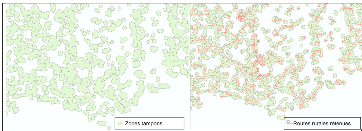
Figure 5 : Exemple de découpage du réseau routier en zone rurale (zone tampon de rayon 250m)
