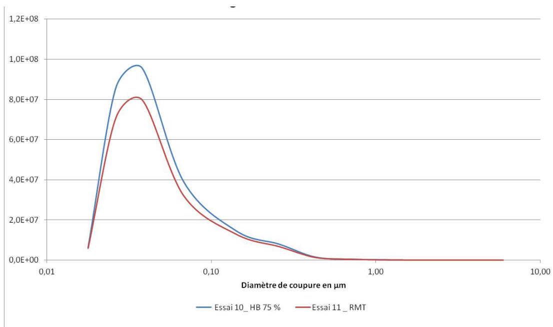
Figure 47 : Distribution granulométrique de la fraction PM 2.5 en fonctionnement ralenti /RMC/HB et RMT, tracteur Massey Ferguson
