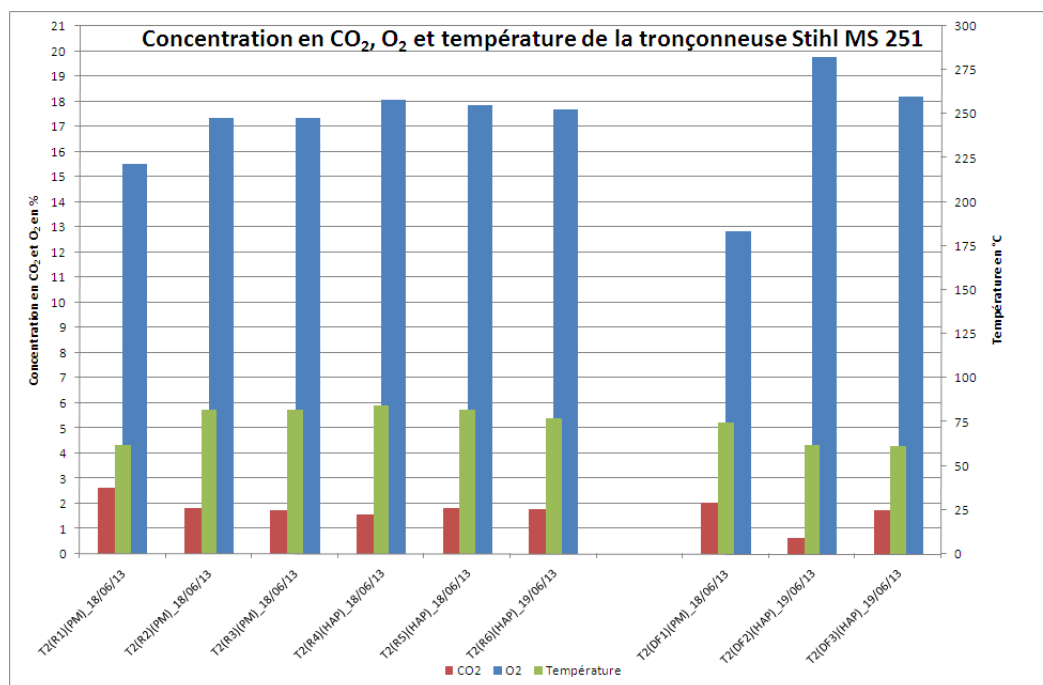
Figure 7 : Comparaison des résultats en CO 2 , O 2 et température pour les différents régimes, tronçonneuse STIHL MS 521
