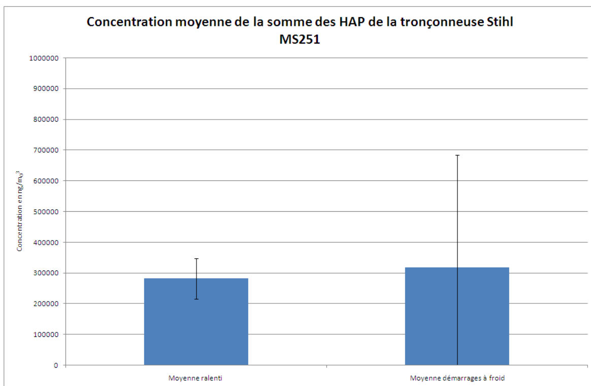
Figure 15 : Comparaison de la concentration moyenne totale en HAP pour les différents régimes, tronçonneuse STIHL MS 521
