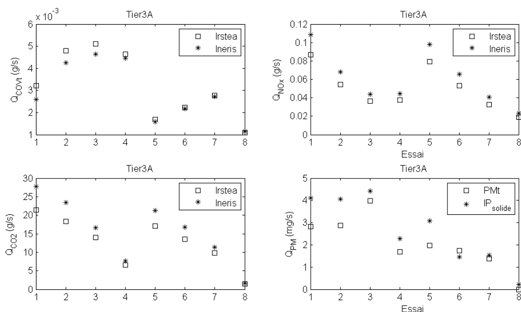
Figure 7- Mesures des débits de polluants mesurés pour le tracteur Massey Fergusson (Tier3A) sur les différents points de fonctionnement
