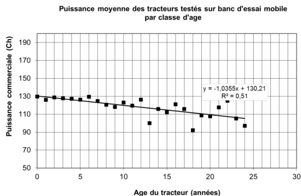
Figure 31 : Evolution de la puissance des tracteurs testés dans le dispositif « banc d'essai mobile » entre 2007-2008 – échantillon de 1200 tracteurs
