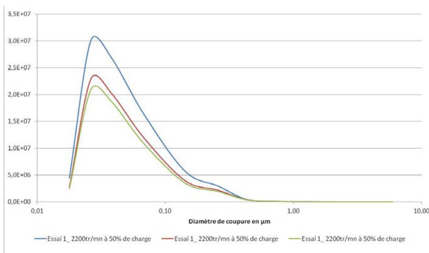
Figure 40 : Distribution granulométrique de la fraction PM 2.5 pour différentes charges à 2200 tour/min, charge à 50%, tracteur New Holland
