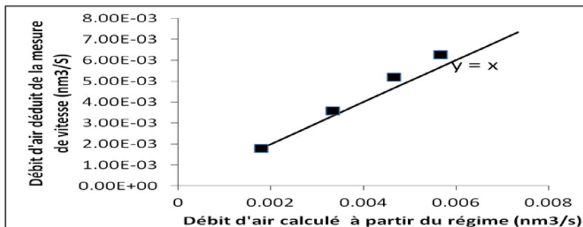
Figure 3 : Comparaison des mesures de débits (nm³/s – 1 bar, 298 °C) par sonde de Pitot et débits estimés à partir du régime moteur
