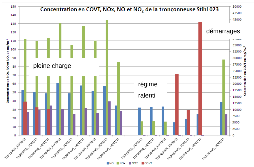
Figure 8 : Comparaison des résultats en COVT, NOx, NO et NO 2 pour les différents régimes, tronçonneuse STIHL 023
