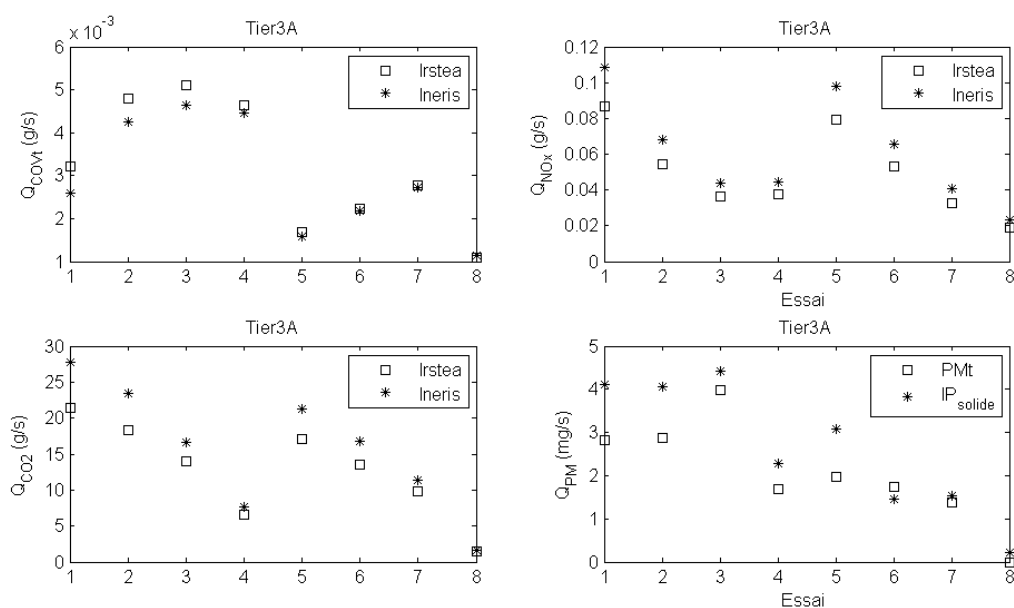
Figure 8- Mesures des débits de polluants mesurés pour le tracteur Massey Fergusson (Tier3A) sur les différents points de fonctionnement
