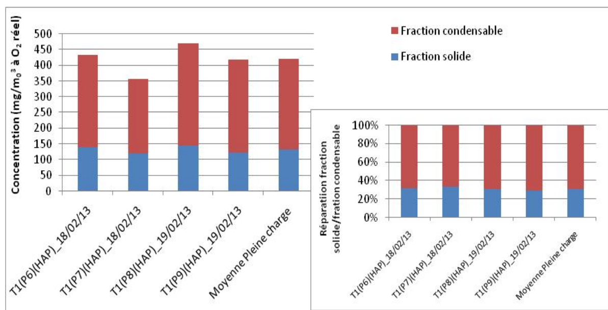
Figure 19 : Répartition de l'aérosol dans les phases solides et condensables, régime ralenti, tronçonneuse STIHL 023
