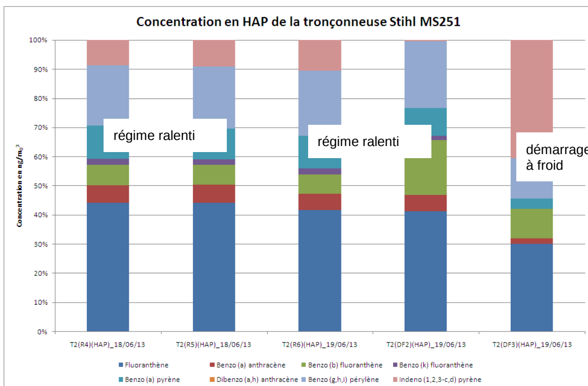
Figure 13 : Comparaison du profil normalisé des HAP pour les différents régimes, tronçonneuse STIHL MS 521
