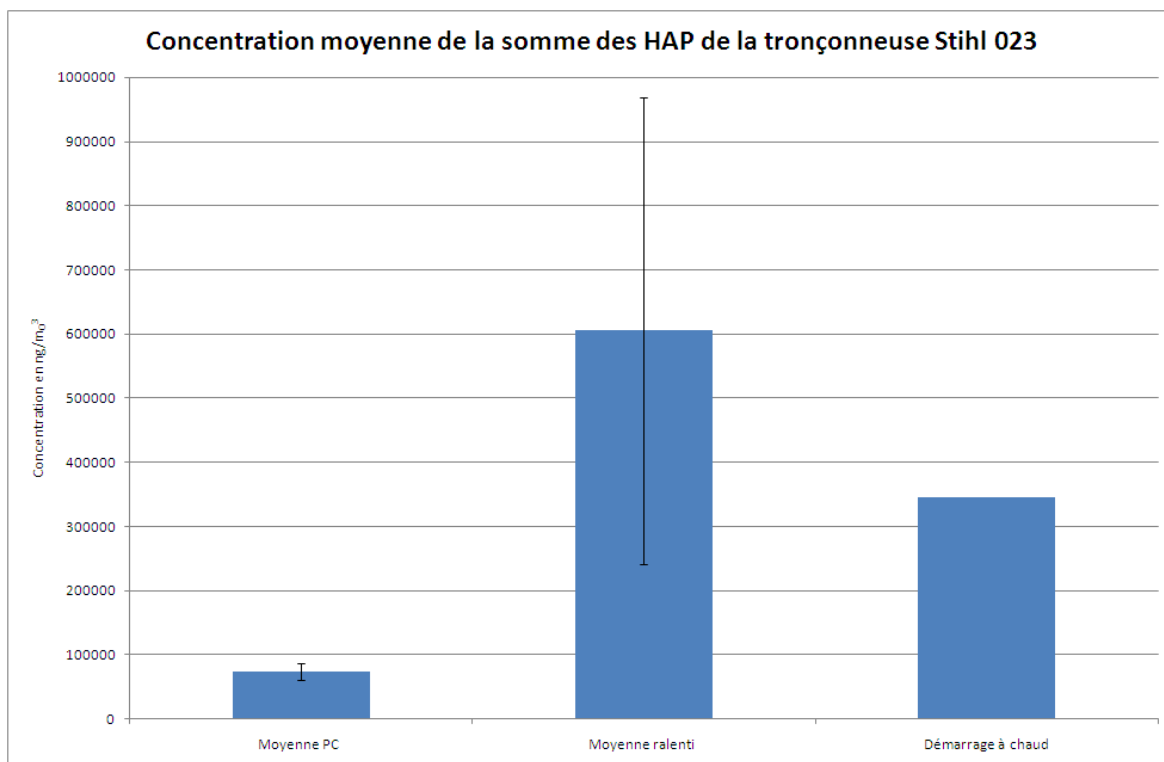
Figure 14 : Comparaison de la concentration moyenne totale en HAP pour les différents régimes, tronçonneuse STIHL 023
