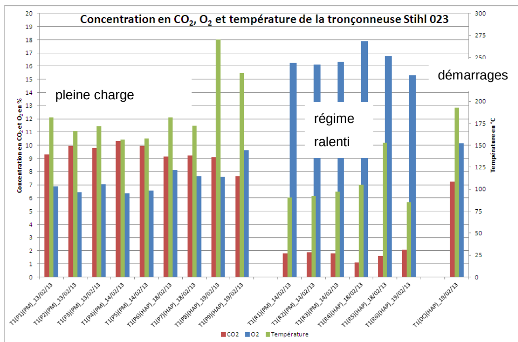
Figure 6 : Comparaison des résultats en CO 2 , O 2 et température pour les différents régimes, tronçonneuse STIHL 023
