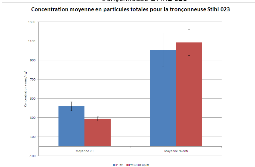
Figure 17 : Comparaison de la concentration moyenne en particules totales pour les différents régimes, tronçonneuse STIHL 023
