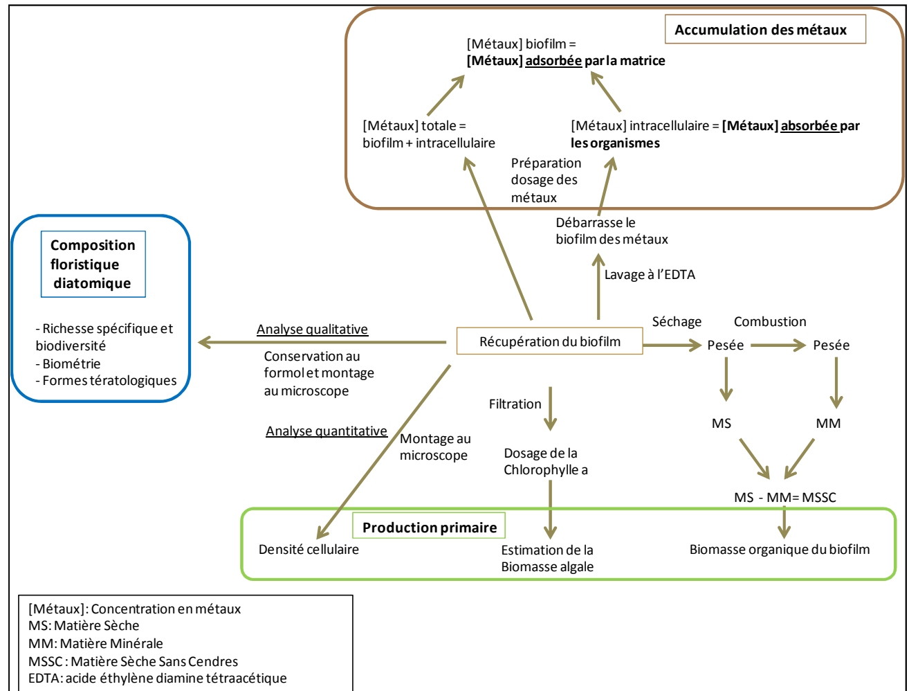
Figure 13, permettant de discriminer la fraction minérale et organique du biofilm. La première étape de séchage déshydrate le biofilm, laissant alors les minéraux et la matière organique desséchée. La phase de combustion volatilise la matière organique laissant seulement la fraction minérale. La différence de masse à la fin des deux phases représente la masse organique.
