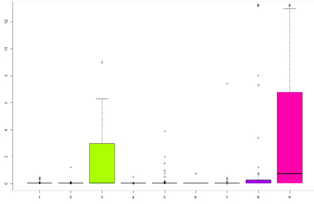
NH4 + (mg/l)
