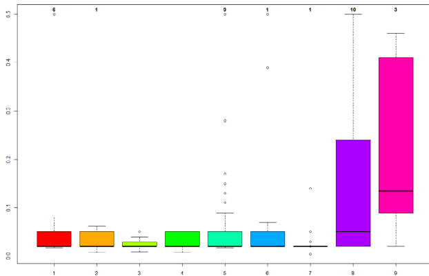
NO2 - (mg/l)
