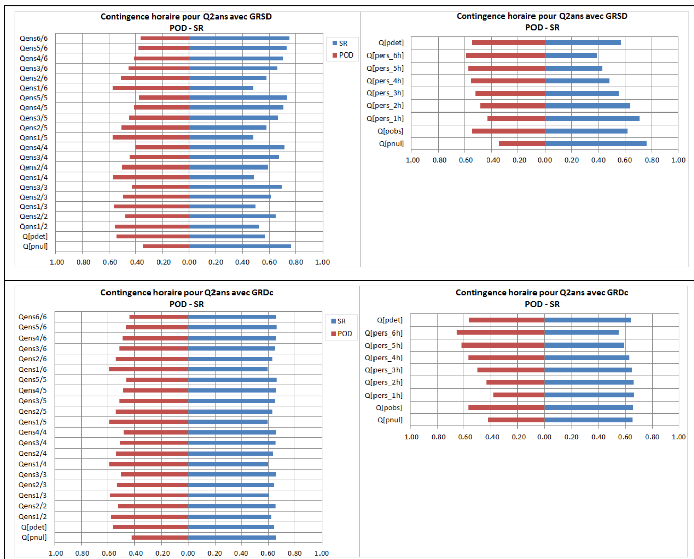
Figure 33 : Scores de Probabilité de Détection (POD) et Taux de Succès (SR) de la contingence horaire avec le modèle semi-distribué (GRSD) et le modèle distribué continu (GRDc) pour le seuil de période de retour de 2 ans
