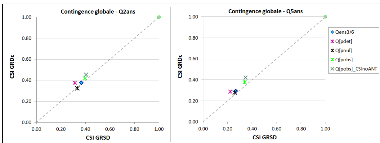
Figure 27 : Comparaison des scores de CSI avec le modèle semi-distribué (GRSD) et le modèle distribué continu (GRDc) pour les seuils de période de retour de 2 et 5 ans
