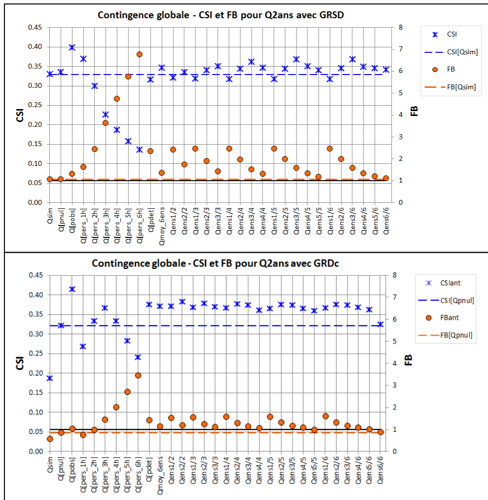
Figure 26 : Scores de contingence CSI (échelle sur la gauche) et de Biases en Fréquence (FB, échelle sur la droite) avec le modèle semi-distribué (GRSD) et le modèle distribué continu (GRDc) pour le seuil de période de retour de 2 ans
