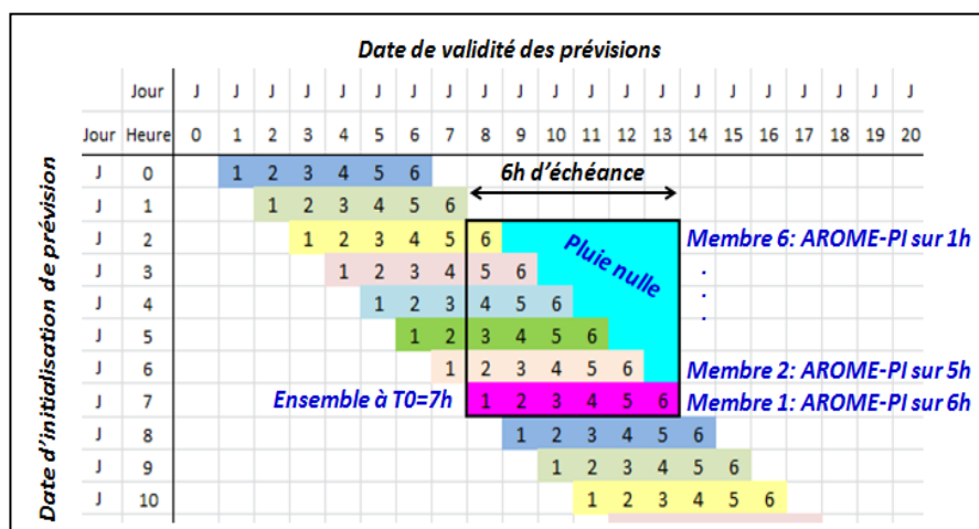
Figure 10 : Schéma de construction des ensembles timelag de pluie à partir des prévisions déterministes AROME-PI successives
