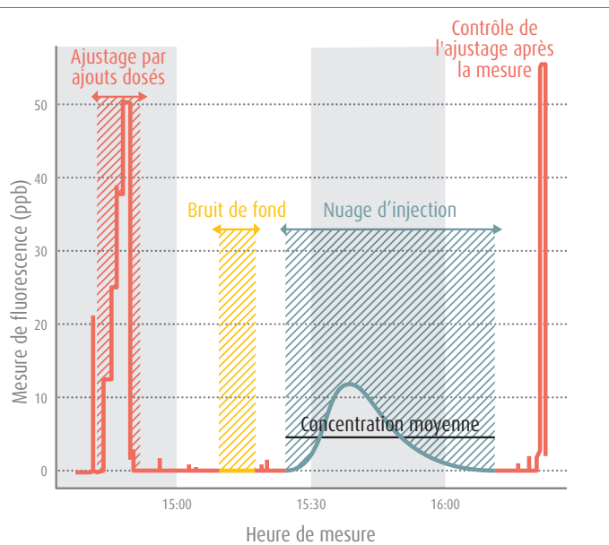
FIGURE 4.13 : À GAUCHE : INJECTION INSTANTANÉE DU TRACEUR RHODAMINE WT ; À DROITE : ENREGISTREMENT DE LA CONCENTRATION AU COURS DES DIFFÉRENTES PHASES DE LA MESURE (AJUSTAGE DES FLUORIMÈTRES, MESURE DU BRUIT DE FOND ET PASSAGE DU NUAGE D'INJECTION), (EDF-DTG)
