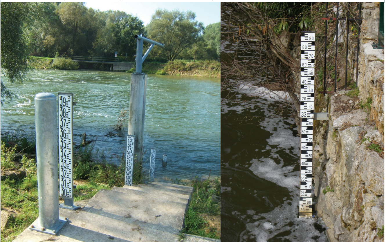
FIGURE 3.1 : À GAUCHE : STATION HYDROMÉTRIQUE À RELATION HAUTEUR-DÉBIT EN SECTION COURANTE, LA MEUSE À STENAY, 3 904 KM 2 (DREAL GRAND-EST, UH MEUSE MOSELLE). À DROITE : ÉCHELLE LIMNIMÉTRIQUE SUR L'YERRES À CROSNES (AQUI' BRIE).
