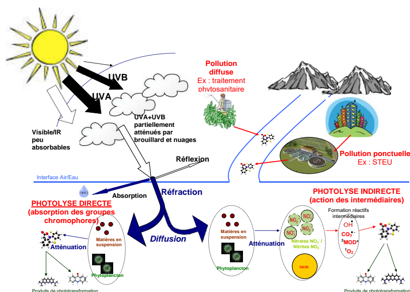
Figure 2 : Représentation schématique de l'action de rayons lumineux sur des molécules organiques contenues dans l'eau (d'après Mathon, 2016)
