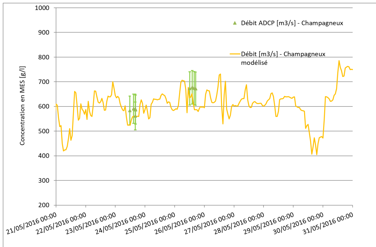
Figure 22 : Variations du débit sur le site de Champagneux
