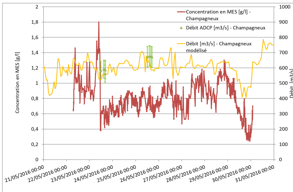
Figure 23 : Variations de concentration en MES et débit à Champagneux
