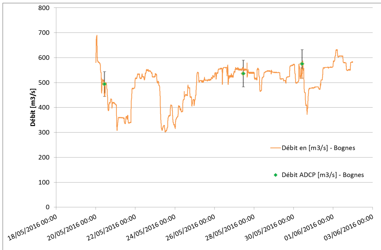
Figure 13 : Variations du débit à la station de Bognes
