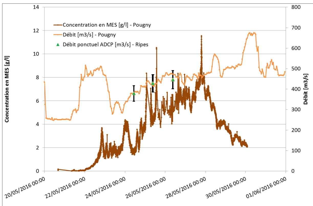
Figure 2 : Variations de concentration en MES et débit à la station de Pougny
