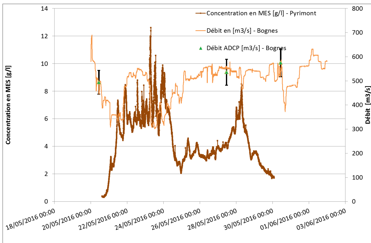
Figure 14 : Variations de concentration en MES à Pyrimont et de débit à Bognes
