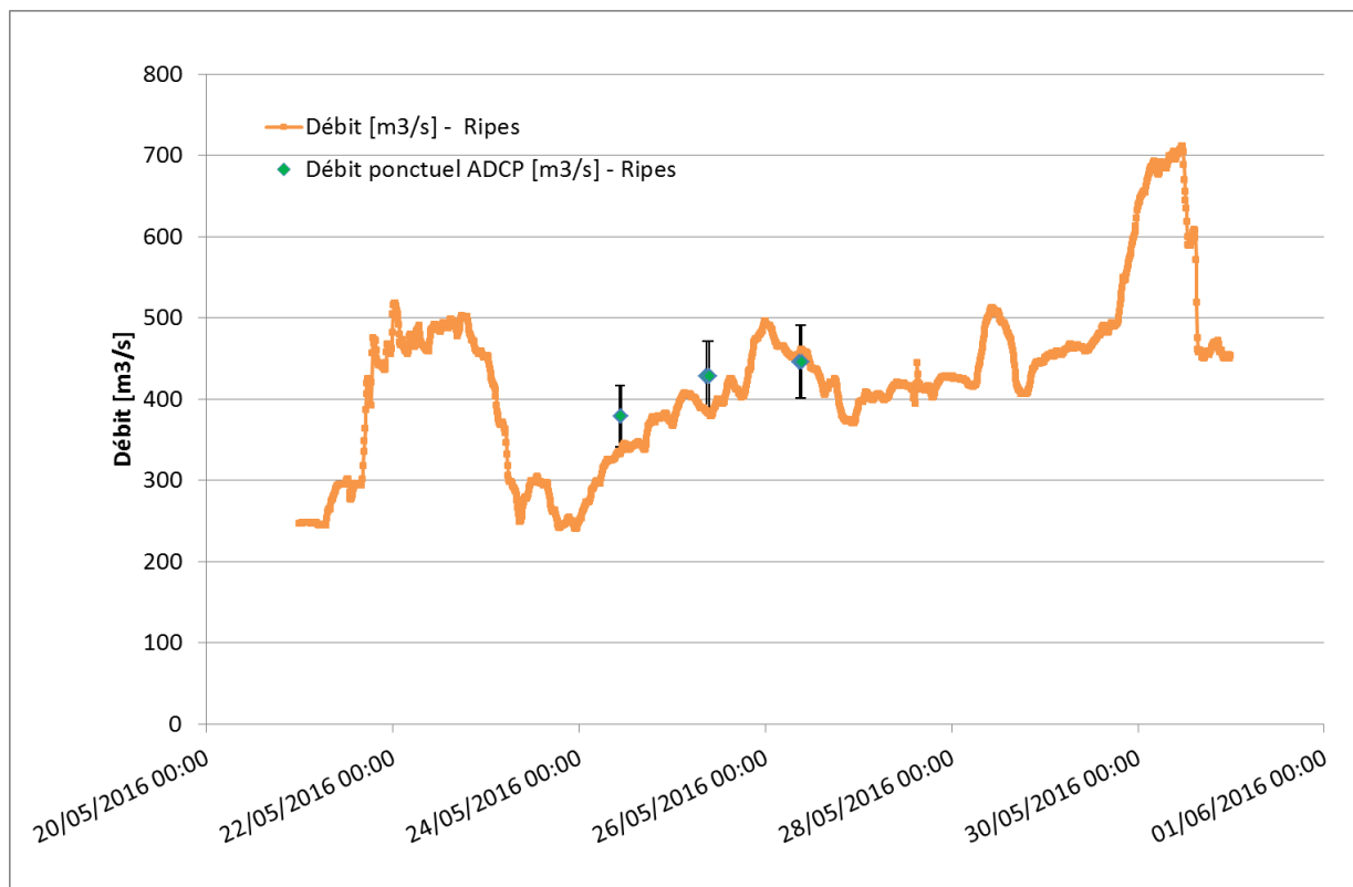
Figure 1 : Variations du débit à la station des Rippes (données OFEV, non validées)
