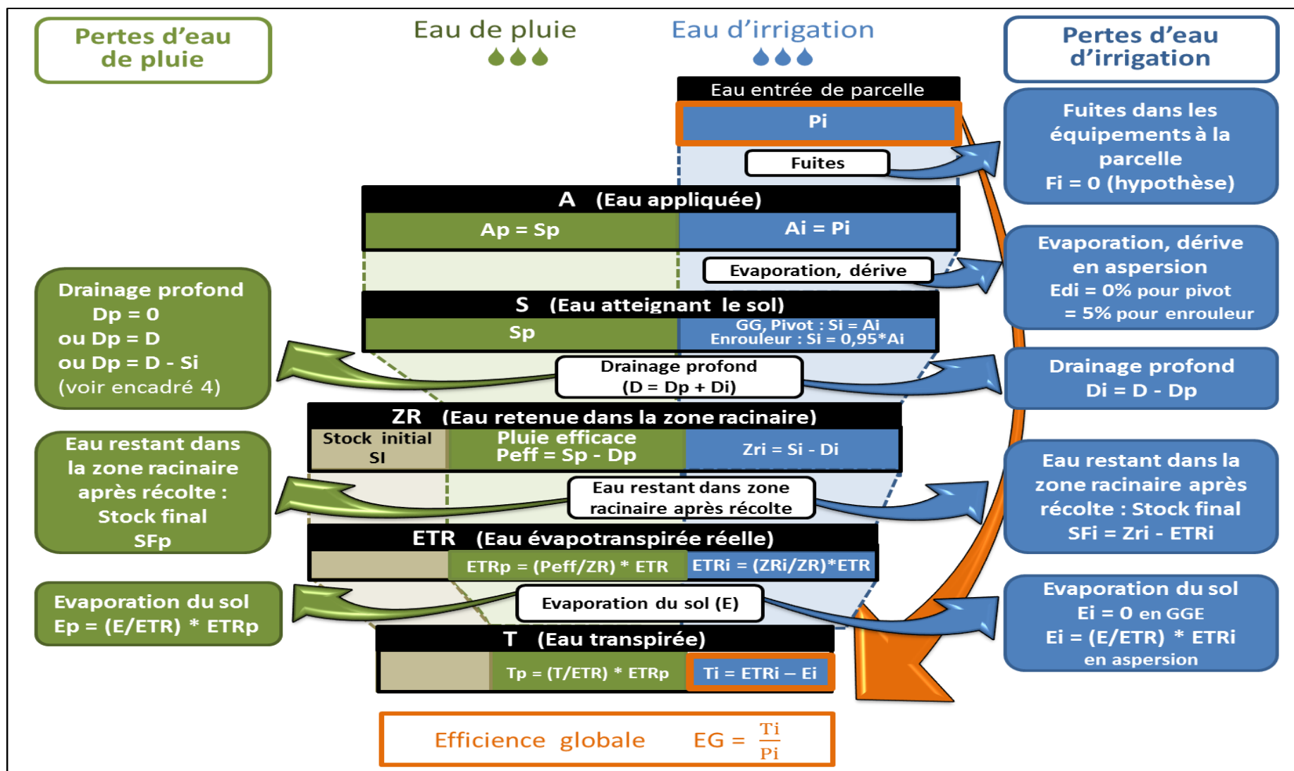
Figure 6. Calcul des volumes d'eau en jeu dans l'efficience globale de l'irrigation
