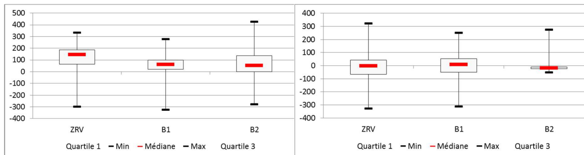
Figures 12 : Comparaison des bilans hydriques sur la ZRV, le B1 et le B2, à débit Q1, à gauche (n = 183) et à débit Q2, à droite (n = 128)
