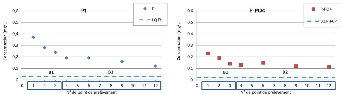
Figure 46 : Evolution des concentrations en phosphore au cours de la ZRV (bilan 24h Irstea du 15 octobre 2015)
