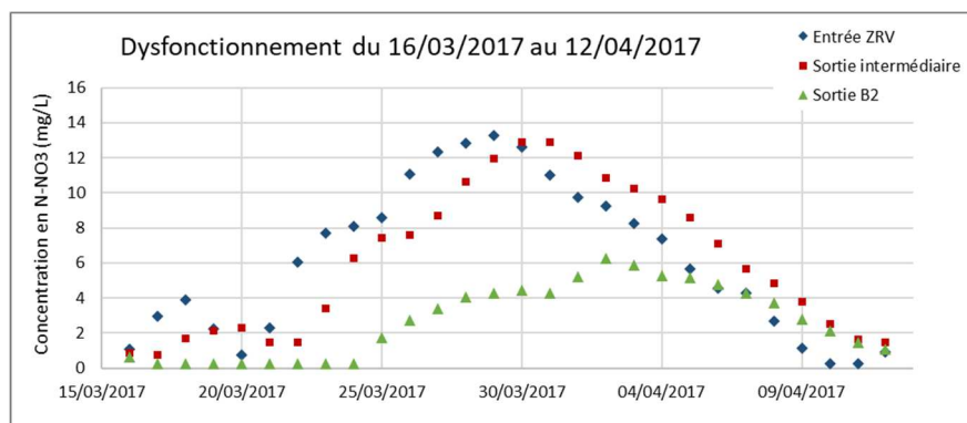
Figure 36 : Evolution des concentrations en N-NO 3 - d'entrée ZRV et sorties mesurées par les sondes (moyennes journalières) lors d'un dysfonctionnement de la station en mars 2017 (charges non calculables car données de débits absentes)
