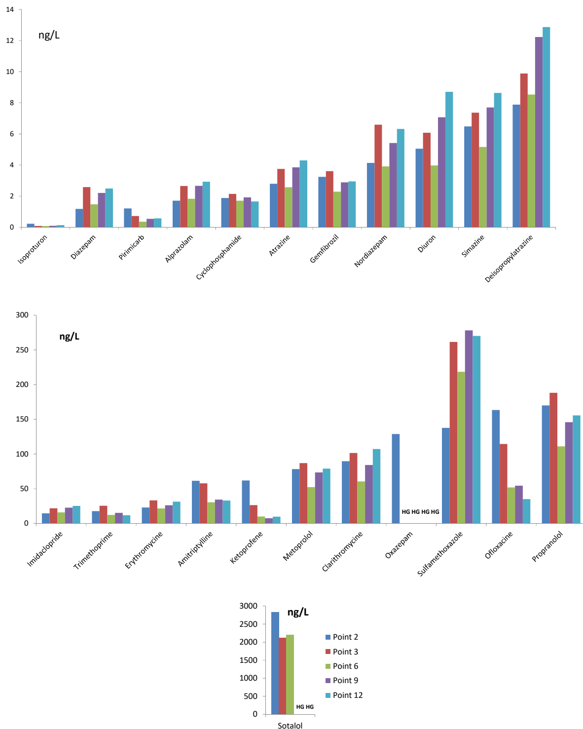
Figure 56 : Concentrations en micropolluants organiques recalculées dans l'eau (ng/L) après échantillonnage par POCIS, en 5 points (entrée ZRV-Point 2 ; sortie B1-Point 3 ; intermédiaire B2 après roselière-Point 6 ; intermédiaire B2 dans zone libre à herbiers-Point 9 et sortie ZRV-Point 12) - Classement par niveaux croissants de concentrations au point 2. HG : hors gamme.
