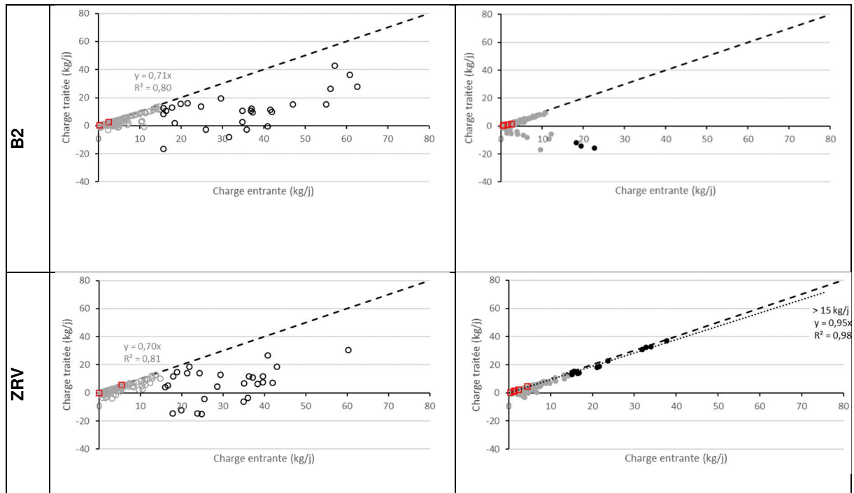
Figure 31 : Charges en N-NH 4 + (données sondes) de janvier 2015 à avril 2017
