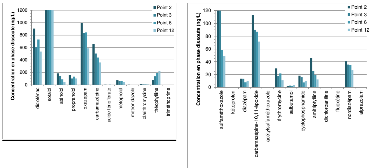
Figure 72 : Concentrations (phase dissoute) en pharmaceutiques mesurées sur les échantillons moyen 24 heures après filtration, en 4 points (entrée ZRV-Point 2 ; sortie B1-Point 3 ; intermédiaire B2 après roselière-Point 6 et sortie ZRV-Point 12) - Classement par famille et par niveaux de concentrations décroissantes (juillet 2015).
