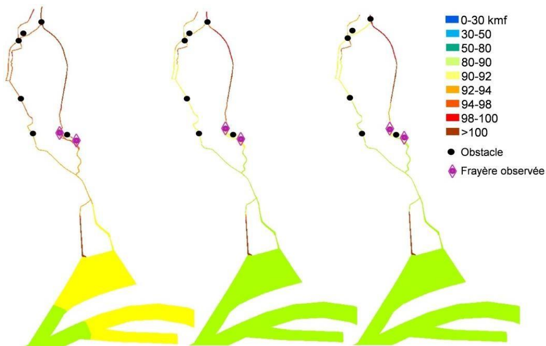
Figure 50. Distances fonctionnelles (kmf) parcourues depuis l'embouchure en fonction des trois coefficients de marée pour le scénario avec le nouveau bras.
