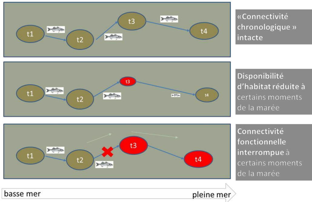
Figure 14. Schéma des effets hypothétiques de la réduction de la disponibilité d'habitat et de l'interruption de la connectivité sur l'accessibilité des nurseries du bar G0 au cours d'une marée. A titre d'exemple, t1-t4 représentent les surfaces d'habitats potentiels à quatre temps successifs de la marée.
