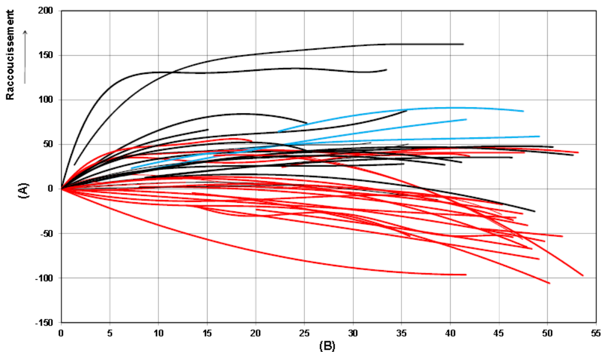
Figure 6 : Analyse menée sur les voûtes EDF en 2003
