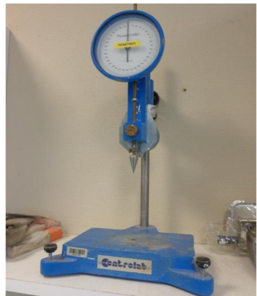
FIGURE 2: CONE DE PENETRATION DE LABORATOIRE
