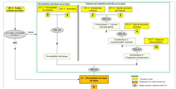
FIGURE 8 : EVALUATION PAR LE MODELE DE LA PERFORMANCE DU CRITERE FONCTIONNEL C1, EI « PERMEABILITE DU CORPS DE DIGUE » A PARTIR DES INDICATEURS D'ETAT DU TRONÇON HOMOGENE DE LA DIGUE RIVE DROITE DU PETIT RHONE, SECTEUR MARIGNAN (IE : INDICATEURS D'ETAT ; C : CRITERES FONCTIONNELS ; EI : EROSION INTERNE)
