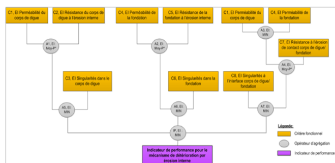
FIGURE 1 : MODELE D'EVALUATION DE LA PERFORMANCE D'UNE DIGUE FLUVIALE VIS-A-VIS DU MECANISME DE DETERIORATION PAR EROSION INTERNE (CI = CRITERE ; EI= EROSION INTERNE ; AI = AGREGATION ; MIN = MINIMUM ; MOY-P* = MOYENNE PONDEREE ; I = INDICE)
