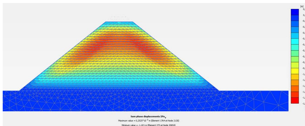
Figure 12 : Déplacements verticaux à 28 mètres de hauteur du barrage en sol non traité, divergence du calcul (PLAXIS).
