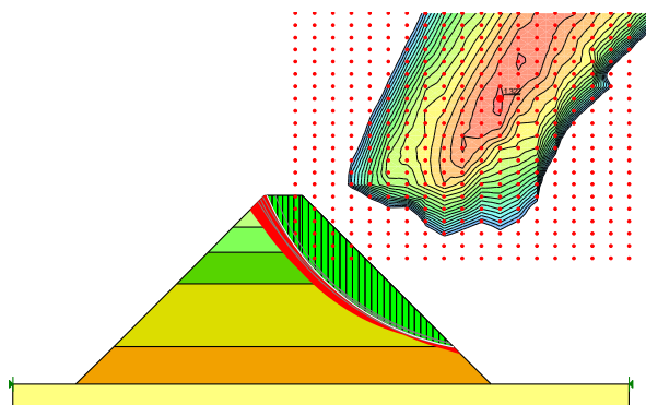
Figure 4 : Facteur de sécurité de 1,32 en fin de construction (pentes 1V/1H - r_u=0,2 avec SLOPE/W). Temps de cure illustrés par des couleurs différentes croissant avec la profondeur des couches dans le remblai.
