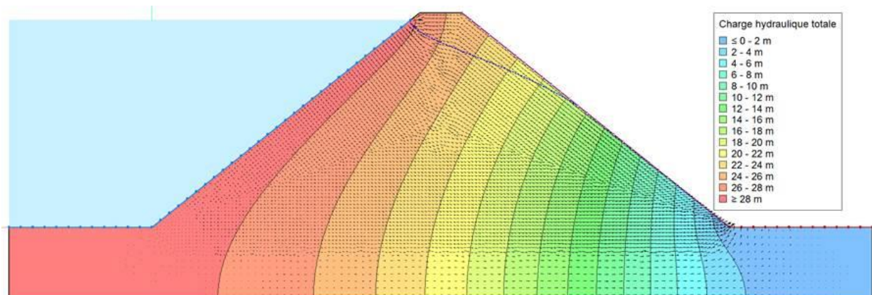
Figure 13 : Niveaux piézométriques en l'absence de masque amont (SEEP)
