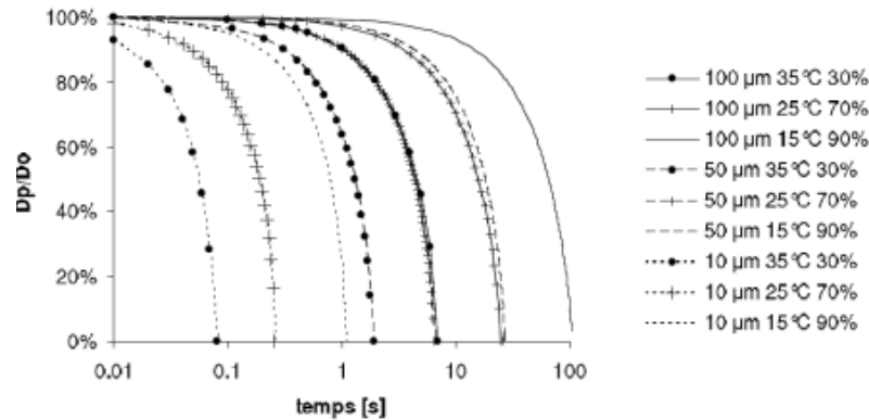
FIGURE 9 : CINÉTIQUES D'ÉVAPORATION DE GOUTTES D'EAU SELON LA TEMPÉRATURE, L'HUMIDITÉ ET LA TAILLE INITIALE DES GOUTTES (D'APRÈS HOLTERMAN, 2003).
