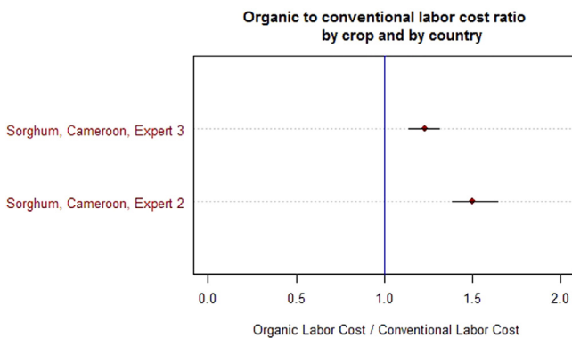
Fig. 4. Médiane et intervalles de crédibilité (80%) du ratio biologique/conventionnel du coût du travail dans la production de sorgho. La ligne bleue représente le seuil pour lequel les coûts de main-d'œuvre dans les systèmes biologiques et conventionnels sont identiques. Chaque point indique la médiane de la distribution élicitée.
