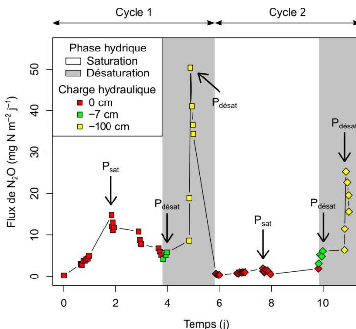
Figure 2 : Évolution des flux de N_2O d'un échantillon de sol au cours de deux cycles de saturation/désaturation ( P_{sat} : pic de N_2O au moment de la saturation en eau, P_{désat} : pic de N_2O au moment de la désaturation en eau).
