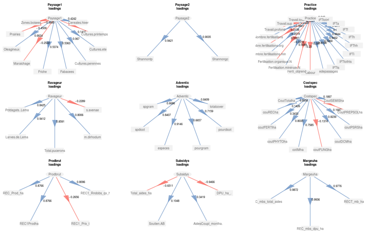
Figure 7. Modèle externe initial de la modélisation structurelle
