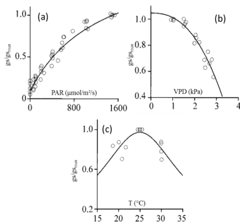
Figure 5: Evolutions caractéristiques de la conductance stomatique normalisée g_s/g_{s,max} en fonction : (a) du rayonnement reçu (PAR), (b) du VPD et (c) de la température foliaire (Pincebourde et al., 2007).
