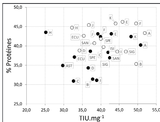
Fig. 2. Relation entre AAT (en TIU par mg) et teneur en protéines sur farine brute sur 15 variétés (une parcelle par variété) observées sur 2 lieux (MON et RIV) en 2014.
