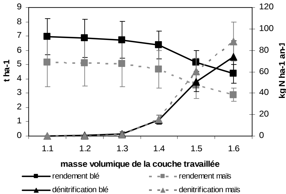
Figure 1. Impact du tassement d'un sol limoneux de Picardie sur les rendements du blé et du maïs (axe de gauche) et les émissions d'azote par dénitrification, en fonction de la masse volumique du sol. Résultats obtenus par simulation avec le modèle STICS. Les barres donnent l'étendue de la variation des valeurs sur la période de référence climatique 1969-2009.
