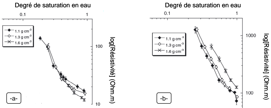
Figure 11 : Résistivité électrique en fonction du degré de saturation en eau pour un échantillon de sol agricole argileux de faible teneur en matière organique (0,7 g.kg -1 ) (-a-) et pour un sol forestier à forte teneur en matière organique (4,2 g.kg -1 ) (-b-). Noter l'échelle logarithmique de résistivité.
