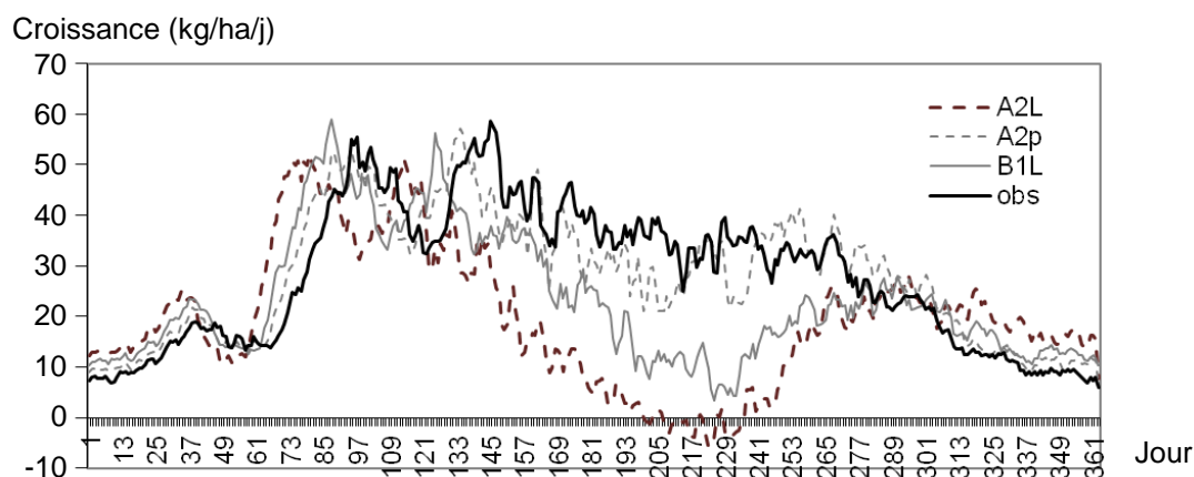
FIGURE 6 – Evolution de la production journalière d'une prairie de graminées en situation actuelle (obs) et dans les 3 séries climatiques (exemple de Pau).
