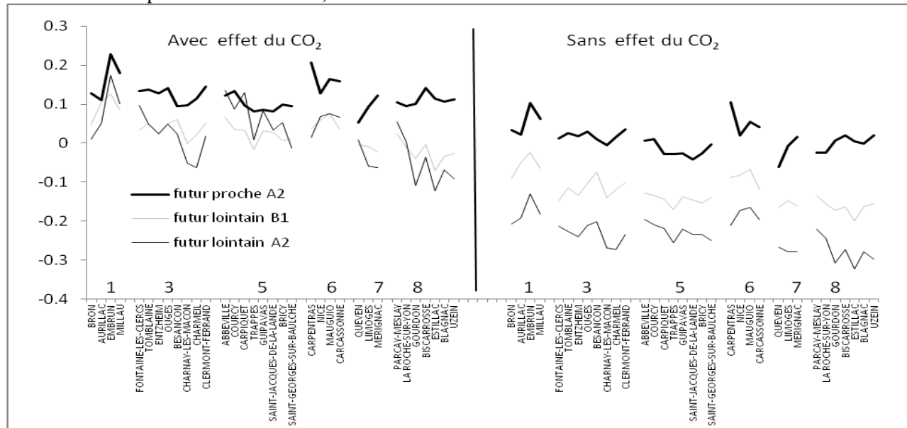
FIGURE 3 – Variations du rendement annuel de la prairie ( par rapport au rendement local présent) par station, pour 3 séries climatiques, avec ou sans prise en compte de l'effet du CO 2 (moyenne sur 27 ans, stations classées par zones de l'AFMS).
