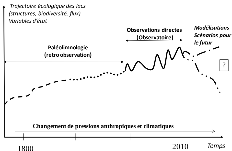
Figure 11 : Schéma conceptuel de l'organisation et de la complémentarité des acquisitions de données environnementales dans le cadre de suivi long terme. Déclinaison adaptée au SOERE Lacs Alpains.(d'après Meybeck et al , 2004).
