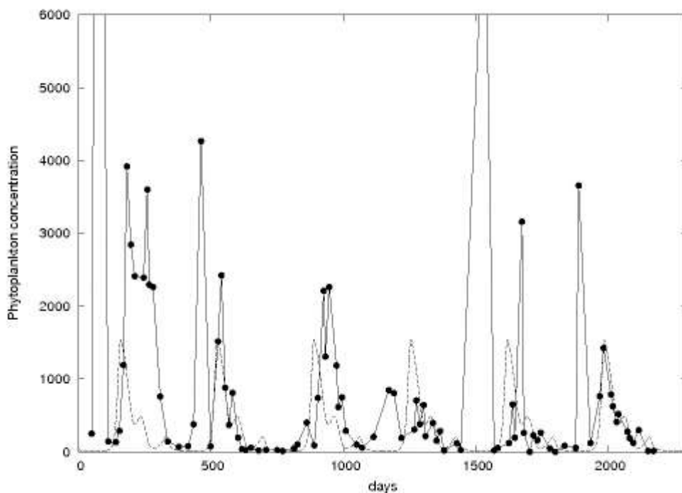
Figure 10 : Concentration mesurée en Chlorophycées (points et traits pleins) et concentration prédite en phytoplancton par le modèle bi couches (lignes pointillées). Les concentrations sont en \mu\text{gC/l} , avec un ratio carbone sur biomasse R = 0,22 . La taille des cellules est estimée à 10\mu\text{m} . Lac Avigliana Grande (d'après Provenzale et Hardenberg, 2012).
