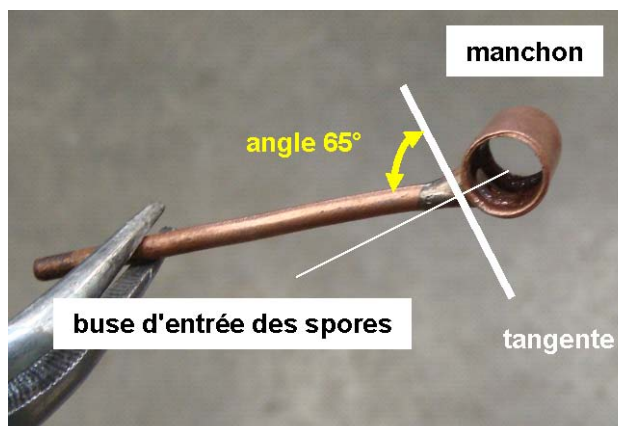
Figure 2. Vue du tube capillaire brasé sur le manchon en cuivre.
