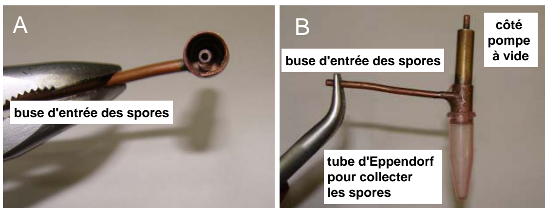
Figure 3. Aspirateur assemblé. A. vue de dessous, côté cyclone, où un tube d'Eppendorf sera emboîté pour récupérer les spores à sec. B. vue d'ensemble avec un tube d'Eppendorf.
