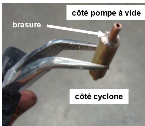
Figure 1. Cœur de l'aspirateur: vue de la brasure du tube en cuivre sur le rondin en laiton.
