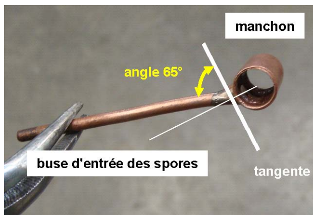
Figure 2. Vue du tube capillaire brasé sur le manchon en cuivre.
