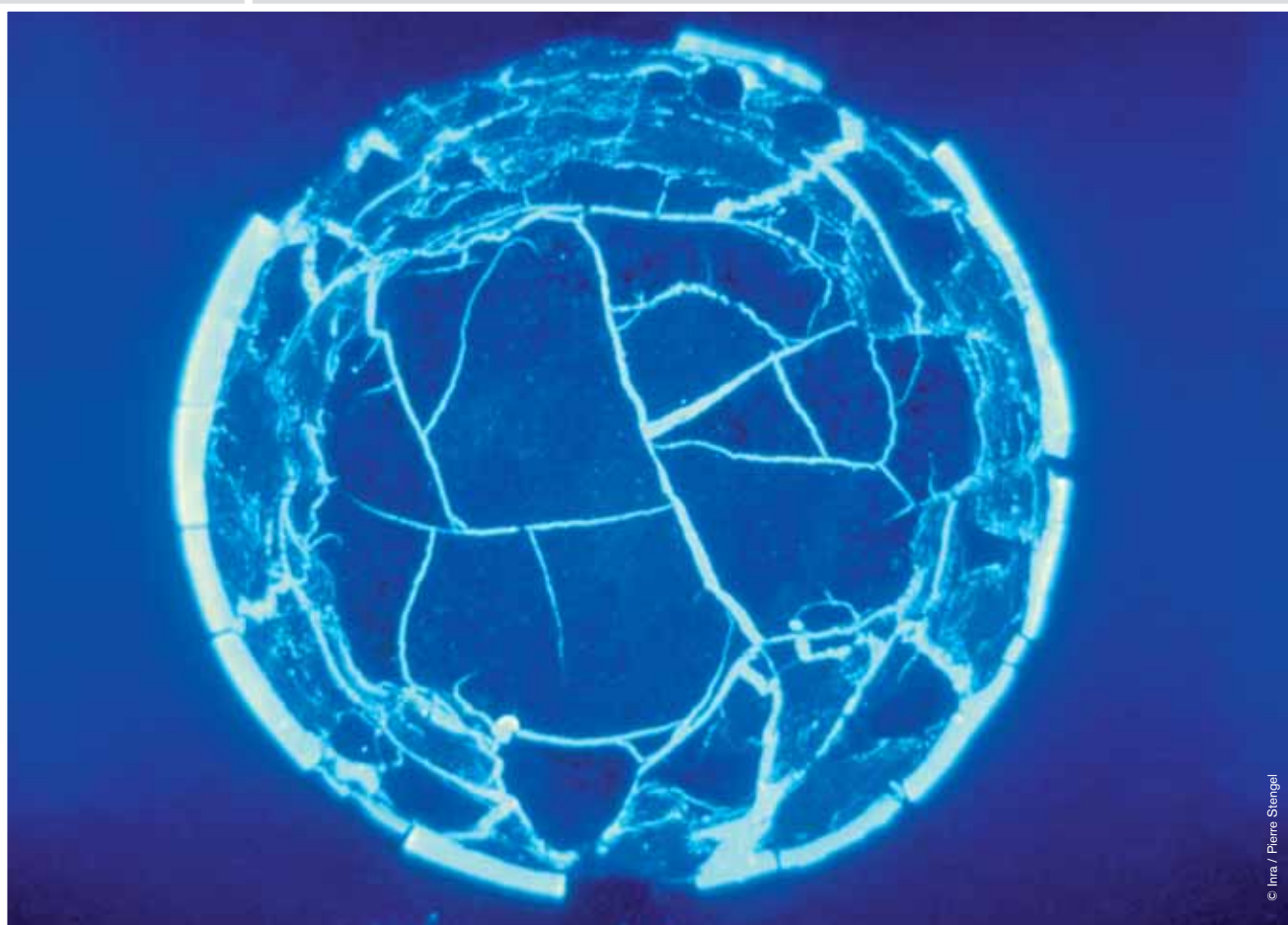
FORMATION DE FISSURES dans un sol argileux en cours d'humectation. Cylindre de terre imprégné par une résine fluorescente et éclairé par ultraviolet.
