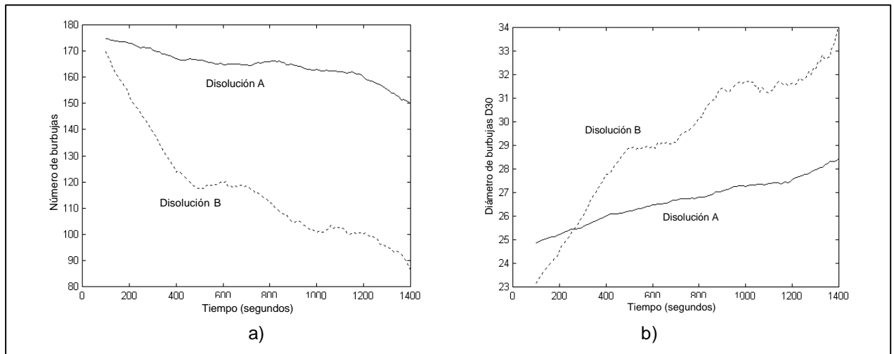
Figura 7. Comportamiento de las espumas en el tiempo, a) Número, b) Diámetro de las burbujas.
