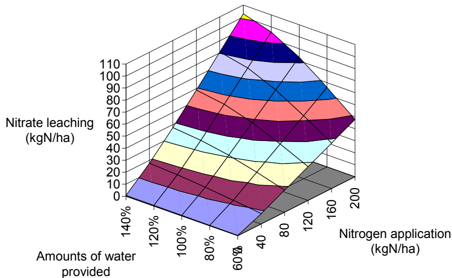
Figure 2 : Relation entre les quantités relatives d'eau et d'azote fournies à la culture et le lessivage de nitrates (de Tourdonnet et al., 2004).
