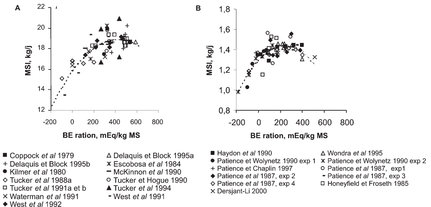
Figure 8. Effet de l'accroissement du BE de la ration sur les quantités de matières sèches ingérées (MSI) des vaches en lactation (A. \text{MSI} = 15,81 + 0,014 \cdot \text{BE} - 1,69 \cdot 10^{-5} \cdot \text{BE}^2 , r^2 = 0,81 , \text{ETR} = 0,996 , P < 0,05 , n = 55 ) et des porcs en croissance et finition (B. \text{MSI} = 1,29 + 0,0012 \cdot \text{BE} - 2,52 \cdot 10^{-6} \cdot \text{BE}^2 , r^2 = 0,98 , \text{ETR} = 0,097 , P < 0,0001 , n = 58 ).
