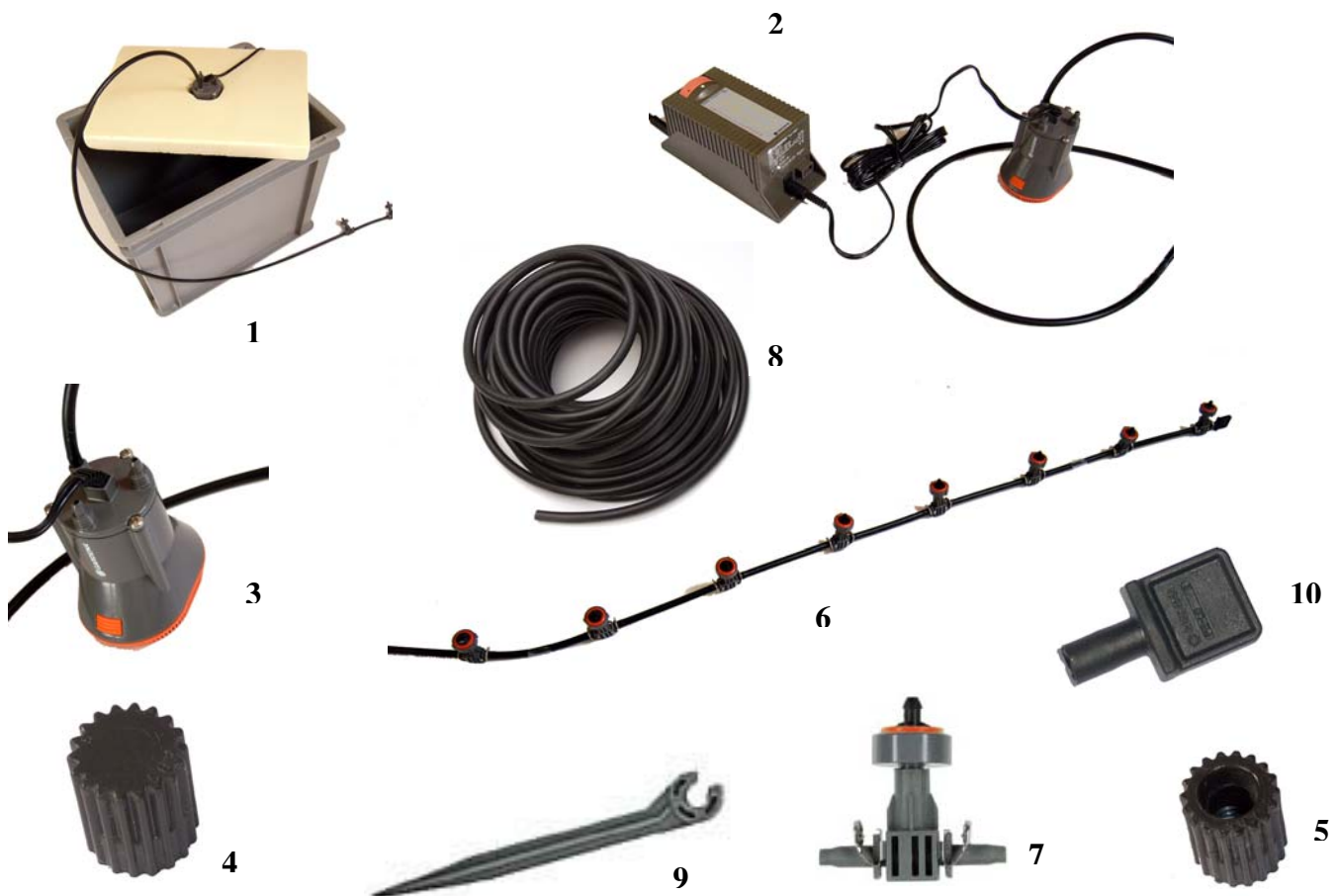
Figure 4 : vue éclatée du dispositif d'arrosage automatique
