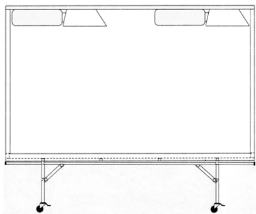
Figure 1 : portique roulant équipé de 2 projecteurs HS 2000 hortilux
