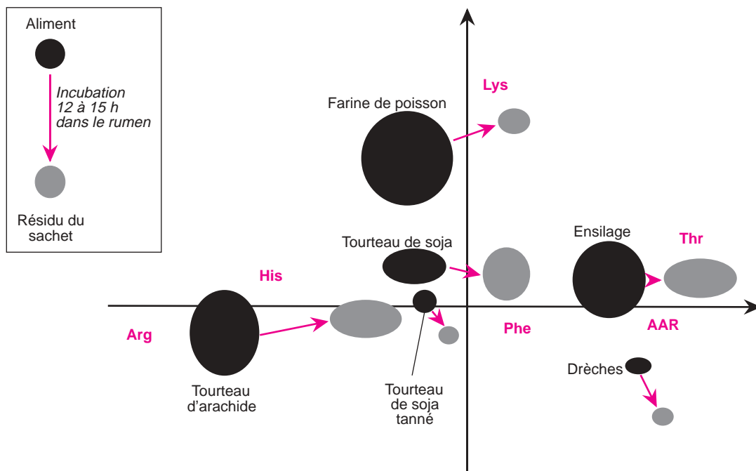
Figure 1. Effets du passage dans le rumen sur le profil en acides aminés des protéines alimentaires (Le Hénaff 1991).
