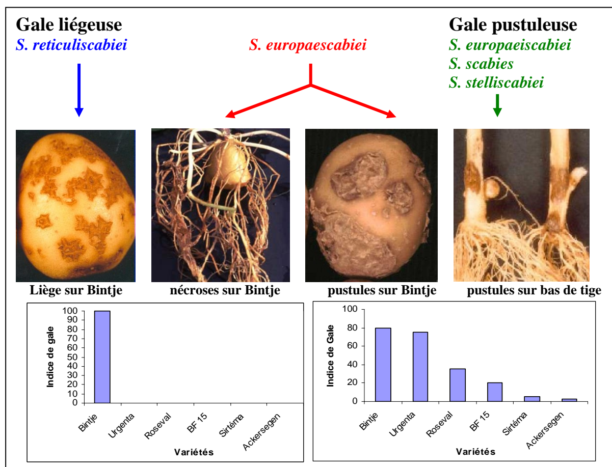
Figure 1 : Différentes espèces de Streptomyces rencontrées en France et description des types de symptômes qu'elles occasionnent sur une gamme de variétés de pomme de terre et de leur sévérité (indice de gale ou IG).
