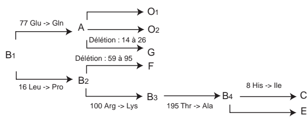
Figure 2. Phylogénie au locus \alpha 1 -Cas chez les caprins.
