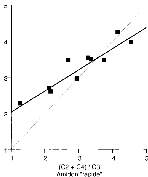
Figure 5. Influence de la nature et de la vitesse de digestion de l'amidon sur le rapport fermentaire (acétate + butyrate) / propionate dans le rumen.
