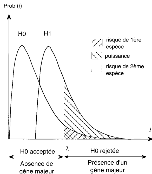
Figure 2. Distributions de la statistique de test l sous H_0 et sous H_1 : définitions des risques de 1ère et 2ème espèces, du seuil de rejet \lambda de H_0 et de la puissance du test. Règle de décision.
