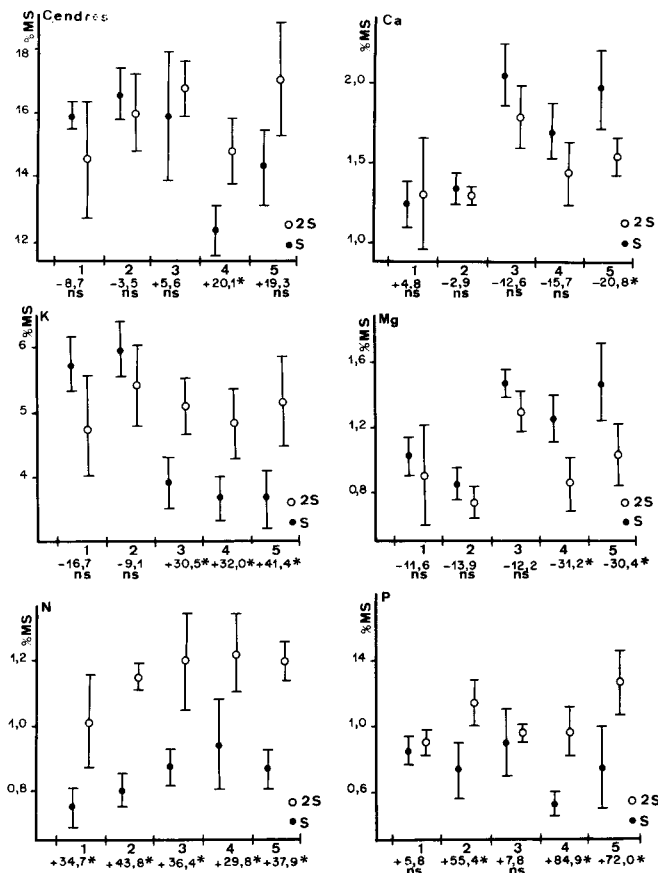
Figure 2 Variation de la teneur (en p. 100 de la matière sèche) des pétioles 1981 en cendres, K, Ca, Mg, N, P (moyenne de 8 plantes et intervalle de confiance au seuil P = 0,05). Porte-greffes : 1 = Rupestris ; 2 = Riparia ; 3 = Fercal ; 4 = 41B ; 5 = 7 542. Le pourcentage d'augmentation ou de diminution de la solution 2S par rapport à la solution S est calculé pour chaque porte-greffe. Le degré de signification statistique est indiqué.
