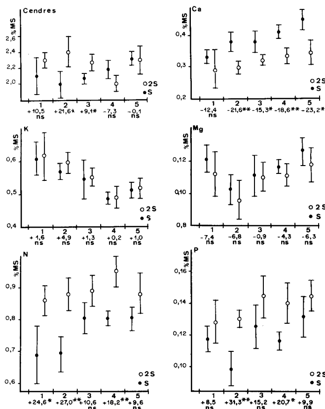
Figure 3 Variation de la teneur (en p. 100 de la matière sèche) des bois 1980 en cendres, K, Ca, Mg, N, P (moyenne de 8 plantes et intervalle de confiance au seuil P = 0,05). Porte-greffes : 1 = Rupestris ; 2 = Riparia ; 3 = Fercal ; 4 = 41B ; 5 = 7 542. Le pourcentage d'augmentation ou de diminution de la solution 2S par rapport à la solution S est calculé pour chaque porte-greffe. Le degré de signification statistique est indiqué.
