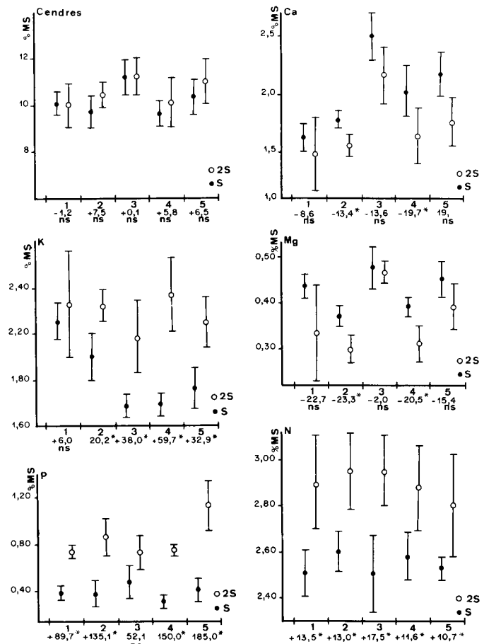
Figure 1 Variation de la teneur (en p. 100 de la matière sèche) des limbes 1981 en cendres, K, Ca, Mg, N, P (moyenne de 8 plantes et intervalle de confiance au seuil P = 0,05 ). Porte-greffes : 1 = Rupestris ; 2 = Riparia ; 3 = Fercal ; 4 = 41B; 5 = 7542. Le pourcentage d'augmentation ou de diminution de la solution 2S par rapport à la solution S est calculé pour chaque porte-greffe. Le degré de signification statistique est indiqué.
