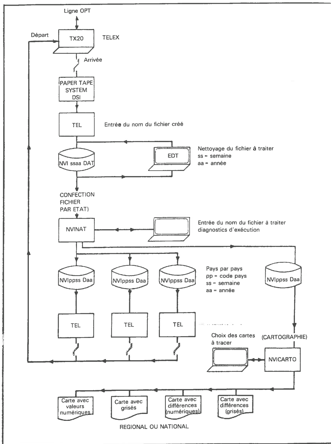
Figure 10. — CHAINE DE TRAITEMENT DES INDICES DE VEGETATION.
