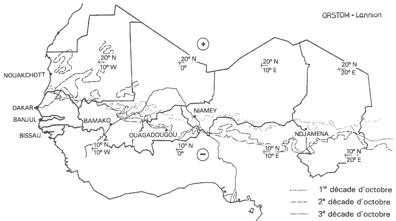
Figure 5. — POSITIONS DE L'ISOTHERME +39°C SUR L'AFRIQUE DE L'OUEST AU COURS DU MOIS D'OCTOBRE.
