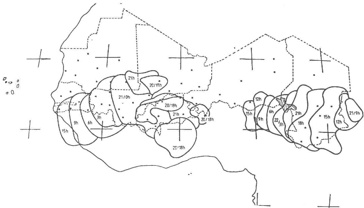
Figure 3. — SUIVI DES AMAS NUAGEUX AYANT INTÉRESSÉ LES PAYS DU CILSS LE 20 ET LE 21 JUILLET 1986.
