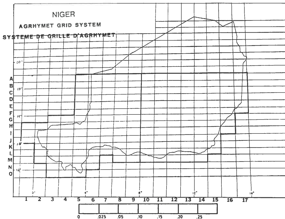
Figure 9. — SYSTEME DE GRILLE D'AGRHYMET.
