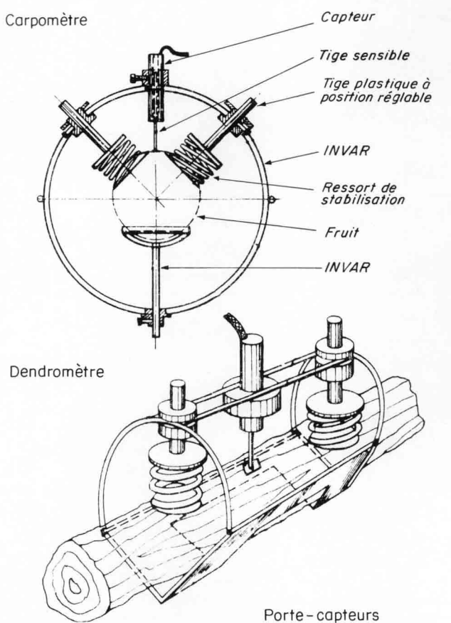
Figure 1 Porte-captteurs de mesure des microvariations de diamètre. Gauge holder for micrometric measurements on fruit (carpometer) and stem (dendrometer).
