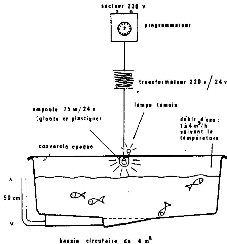
Figure 1 : Exemple d'installation pour le contrôle photopériodique de la reproduction de la truite.
