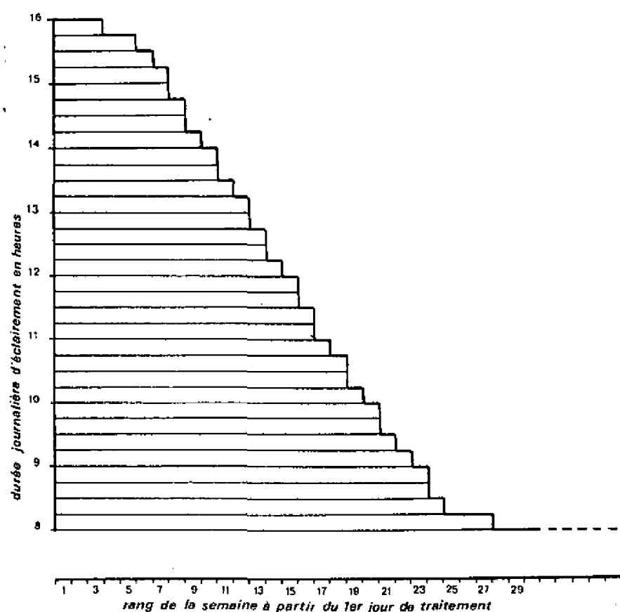
Figure 2 : Exemple de programmation de la durée journalière d'éclairage à appliquer (compte tenu du réglage par 1/4 d'heure des programmeurs du commerce).
