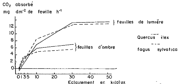
FIG. 2. — Fabrication des assimilats. Assimilation du \text{CO}_2 par une feuille en fonction de l'éclaircissement.
