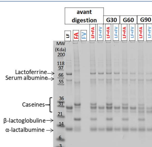
Fig 3. SDS-PAGE
