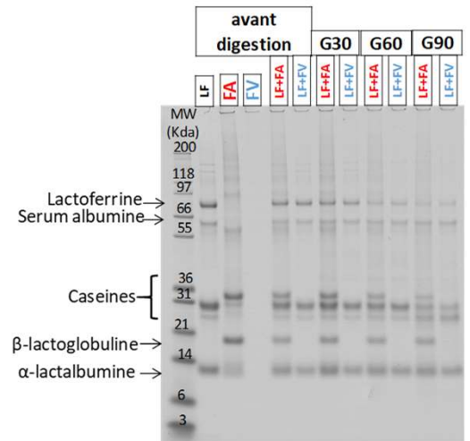
Fig 3. SDS-PAGE
