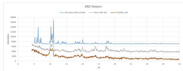
Xrd comparison.png
