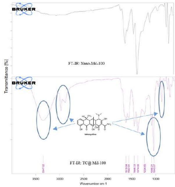
Ft-ir comparison.png
