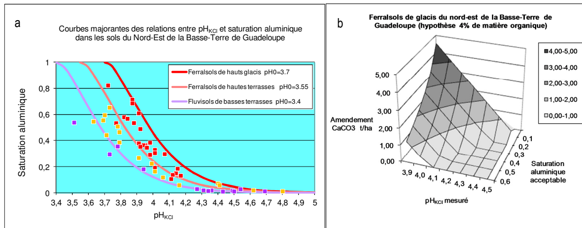
Figure 4 : Utilisation d'une relation caractéristique des sols établie en laboratoire pour raisonner le chaulage d'un ferralsole de Guadeloupe
